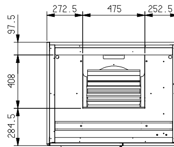
Centrifugal Fan
